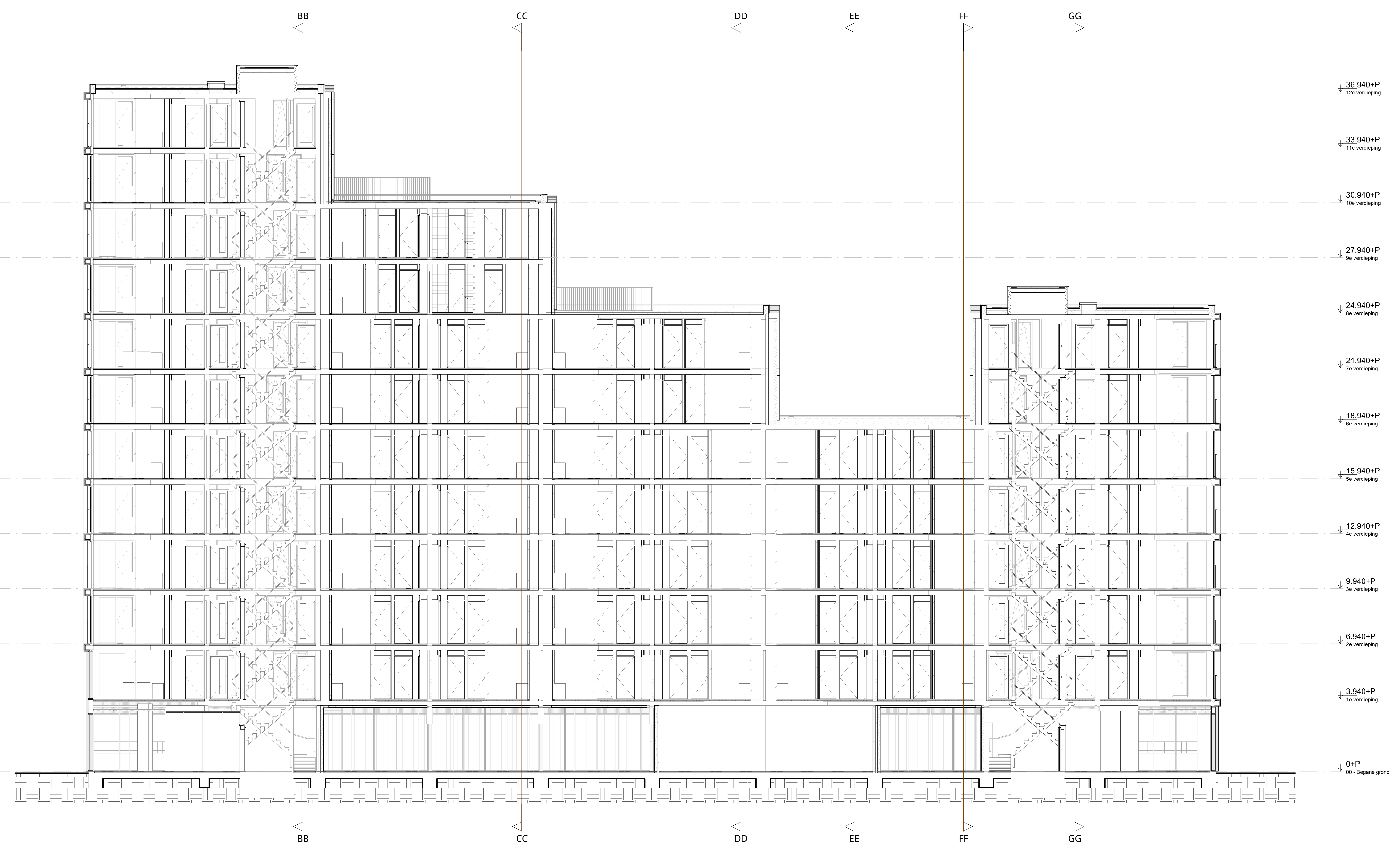
Doorsnede AA
