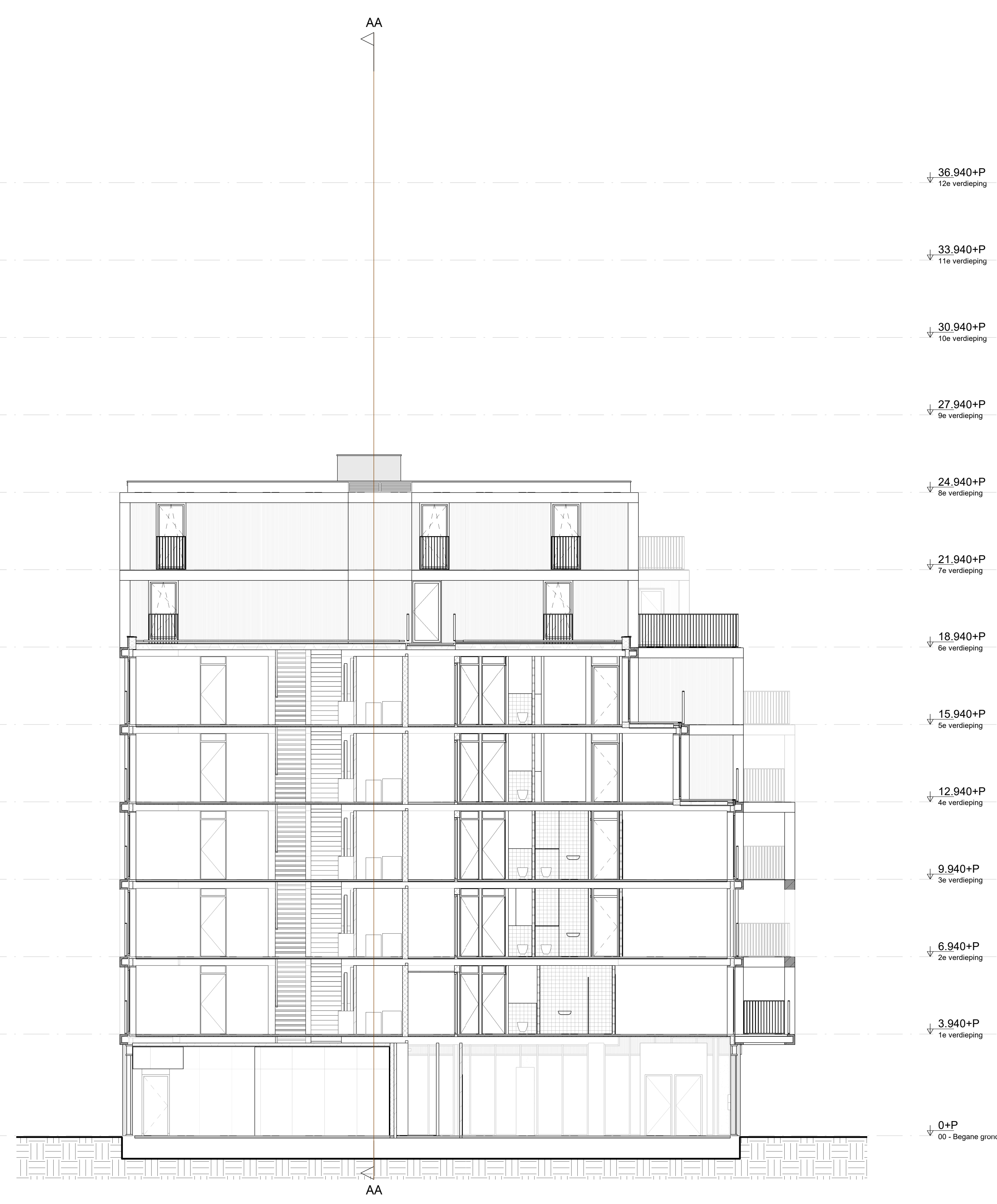
Doorsnede FF
