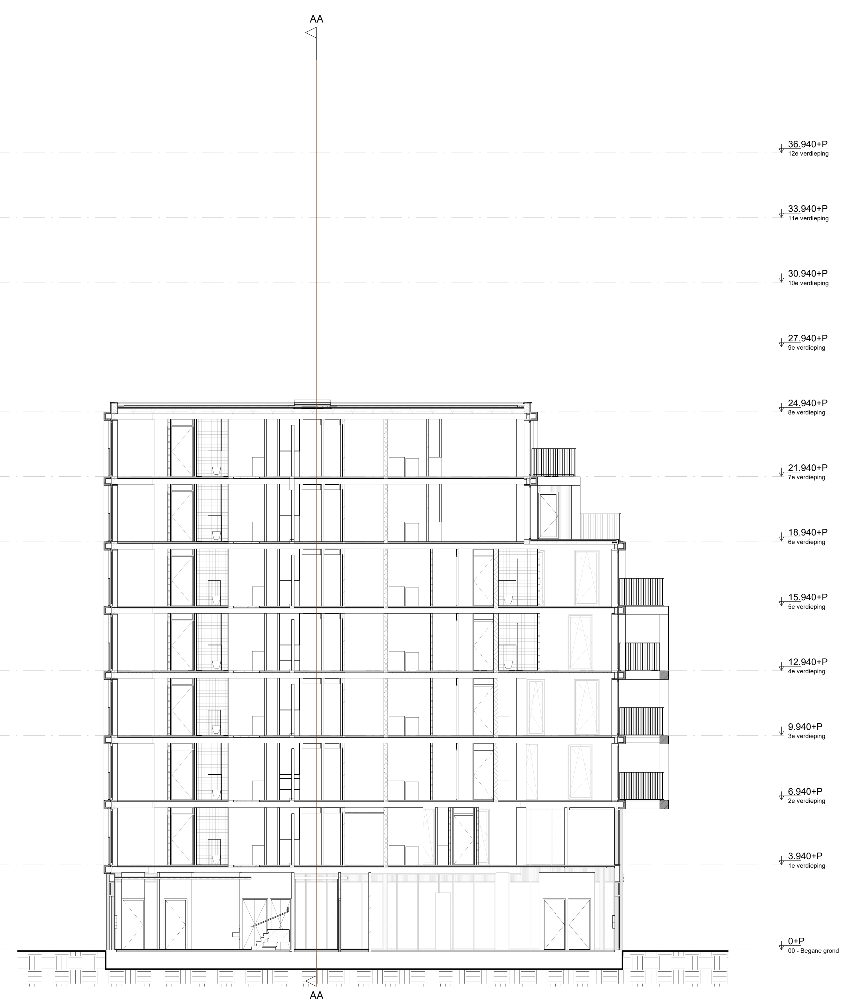
Doorsnede GG
