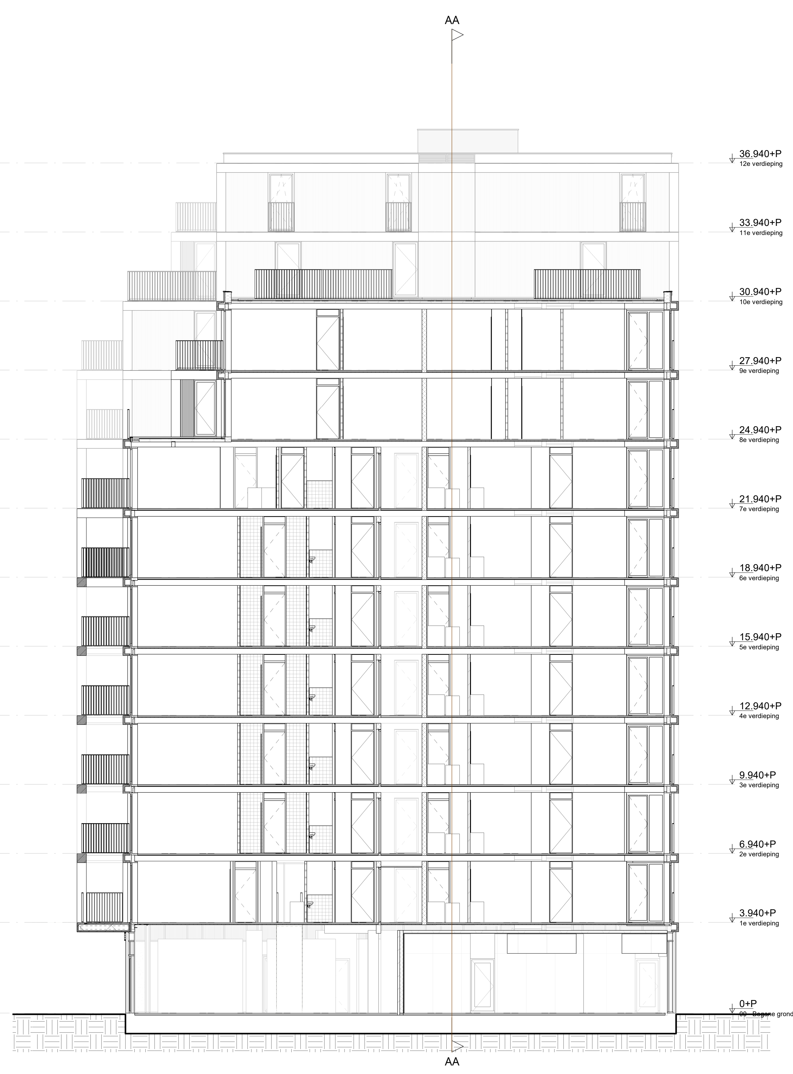
Doorsnede CC
