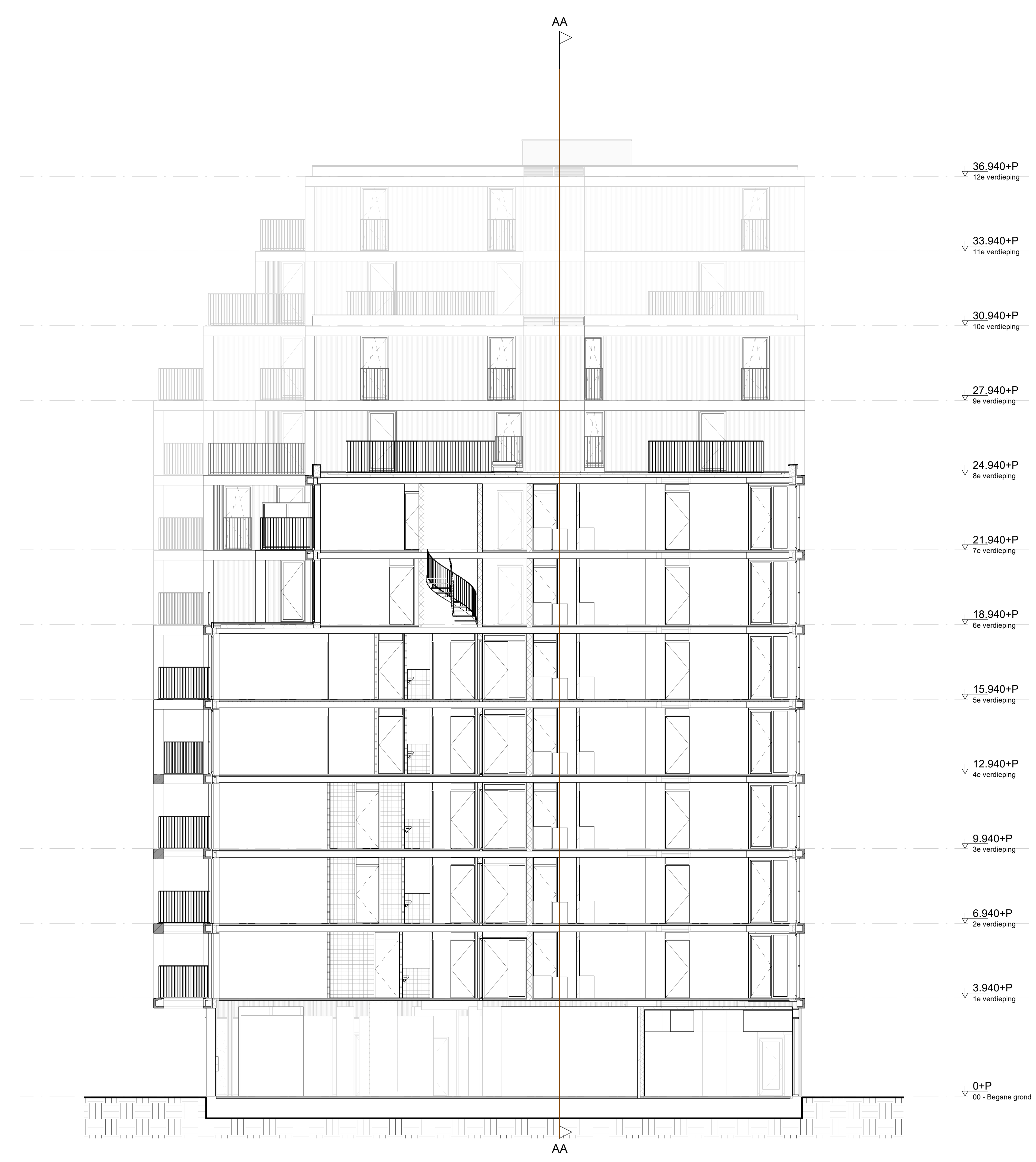
Doorsnede DD
