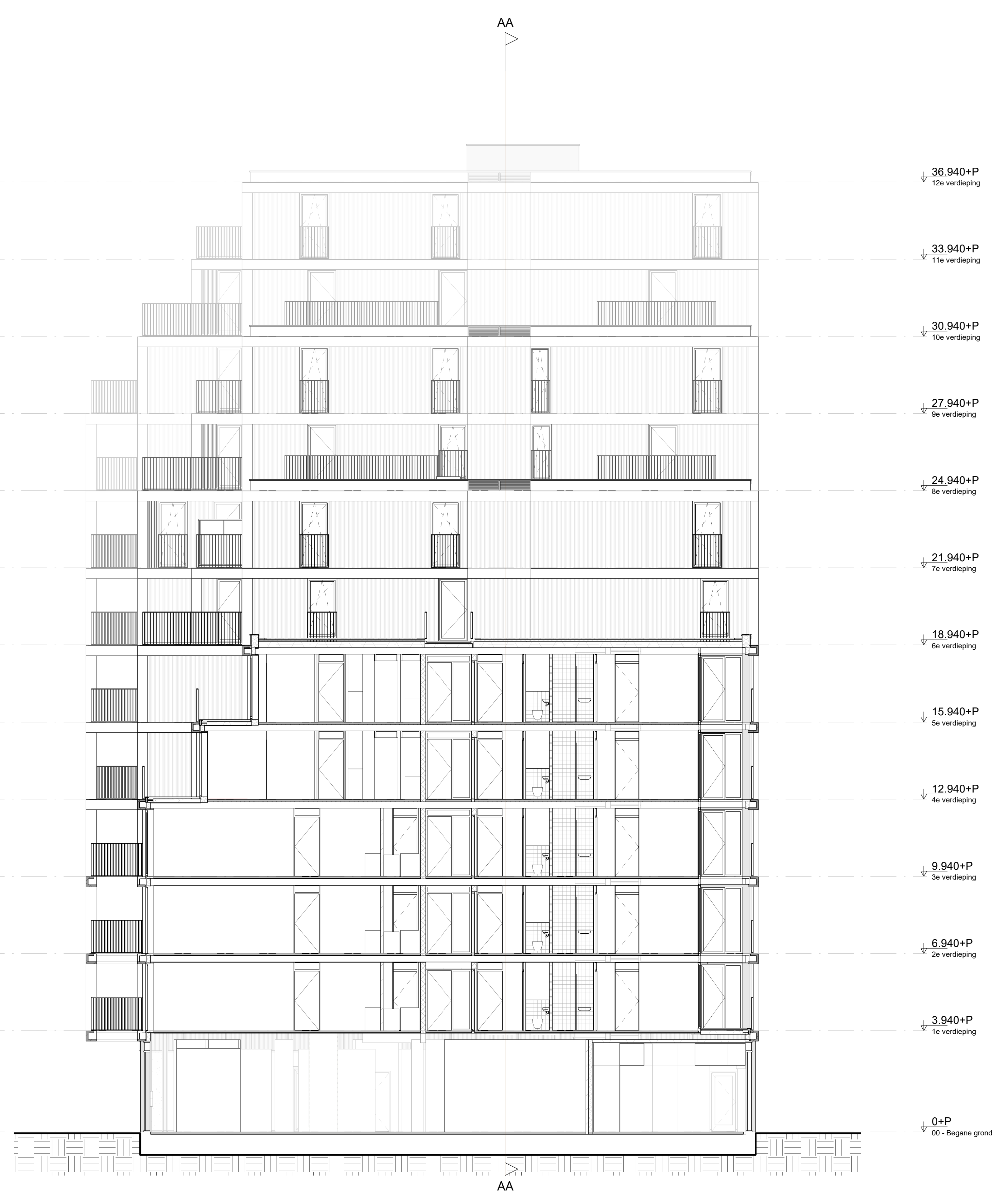
Doorsnede EE
